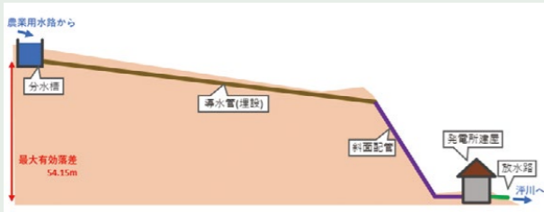
【図1】小水力発電施設
