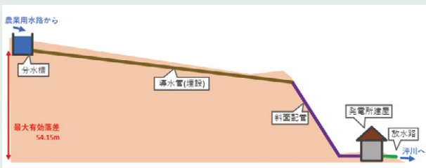
【図1】小水力発電施設
