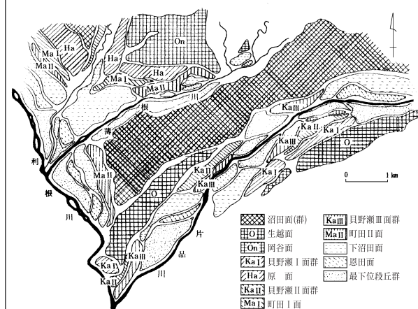
沼田付近に分布する河岸段丘の区分『沼田市史 自然編』(1995)より
