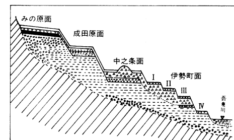
中之条付近の段丘模式断面図(山口原図1975)
