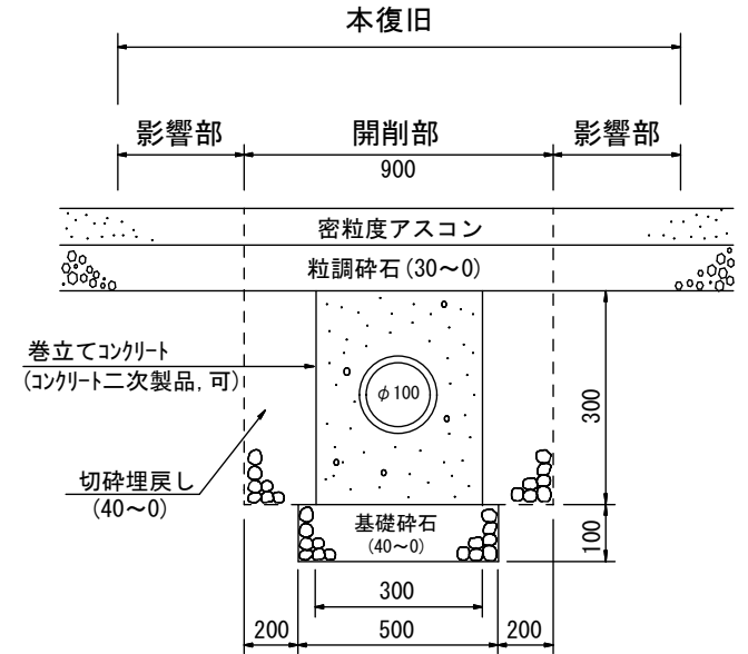
1※ 砂巻き立ての場合の標準断面図
