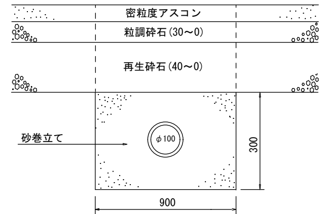
1※ 砂巻き立ての場合の標準断面図
