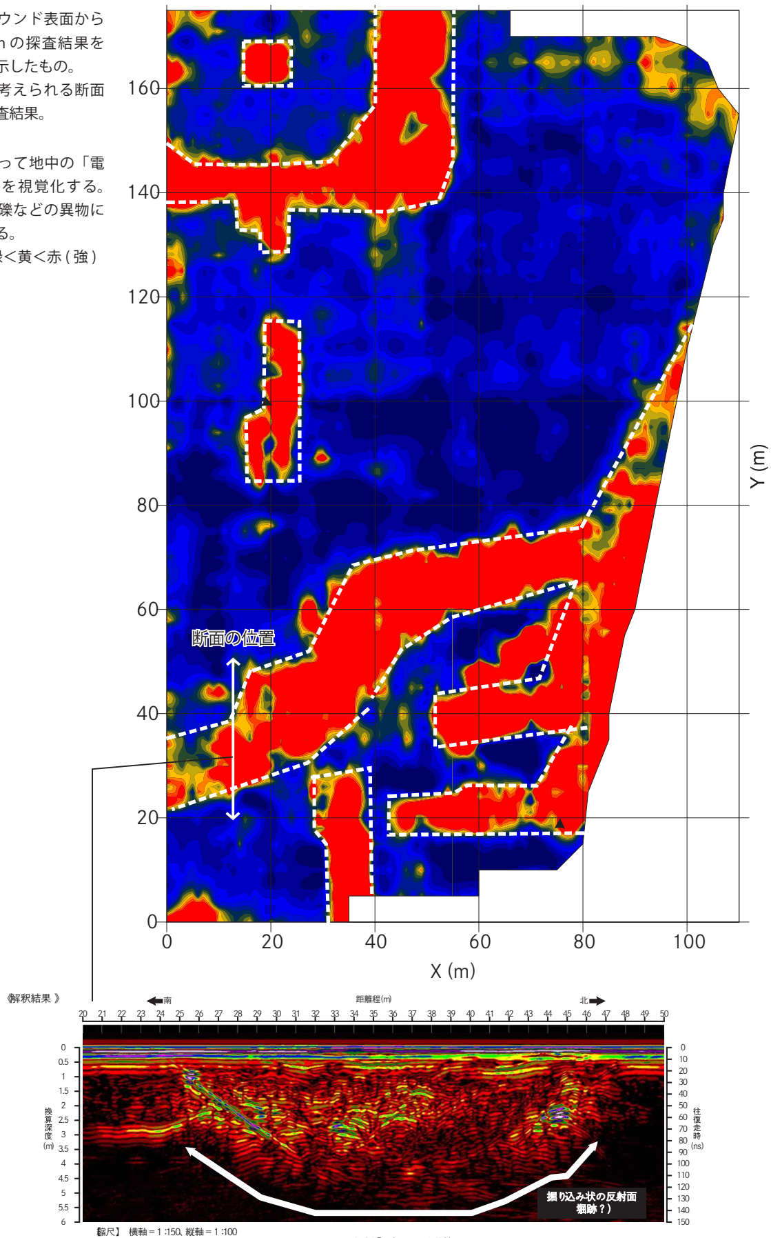
図 3-2 記録例① (X010m測線)
