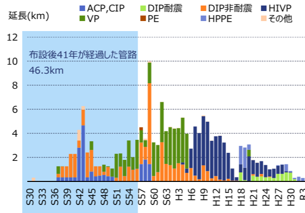
図-3 管路布設延長の推移：上水道
