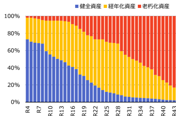
図-16 資産の健全度：簡易水道
