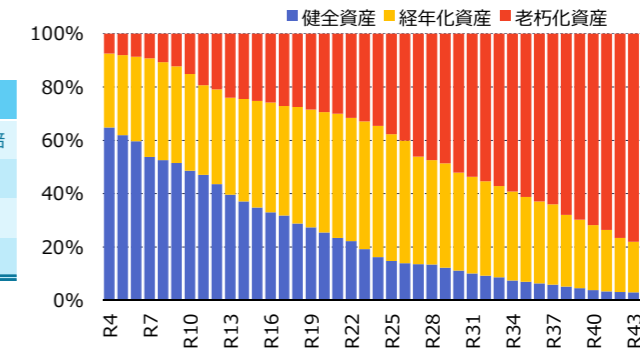
図-13 資産の健全度：上水道
