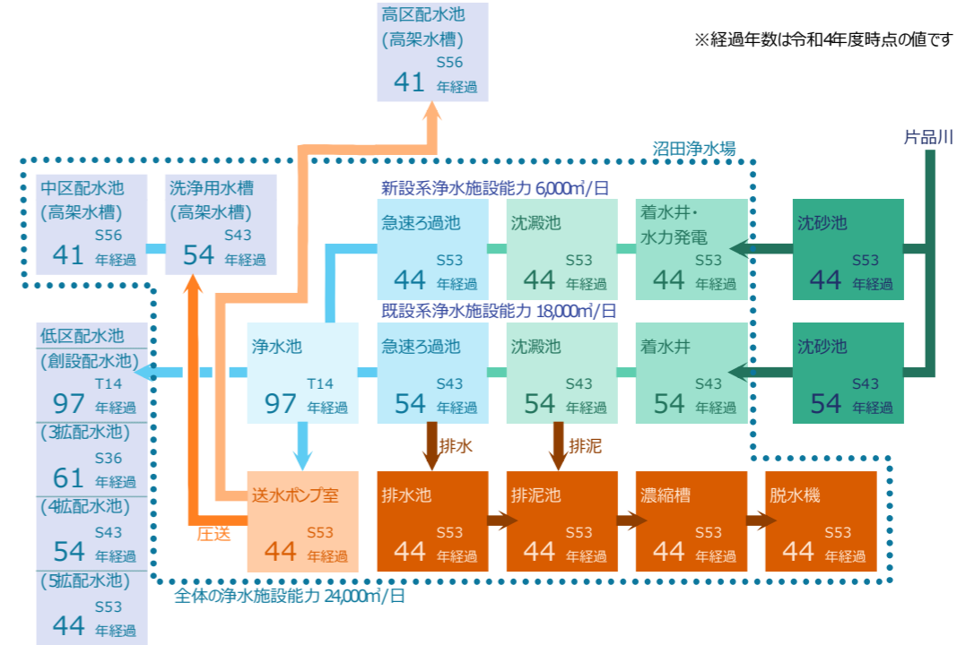
図-4 沼田浄水場 施設フローと経過年数
