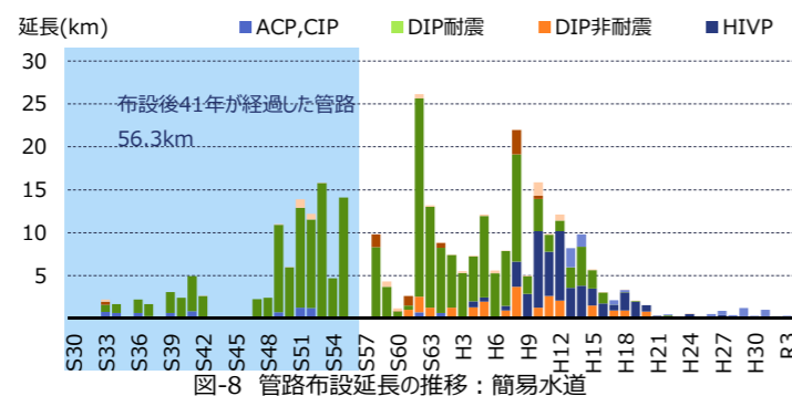
図-8 管路布設延長の推移：簡易水道
