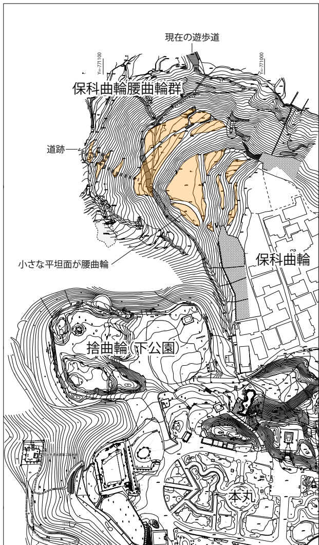
北側段丘崖腰曲輪群測量図
